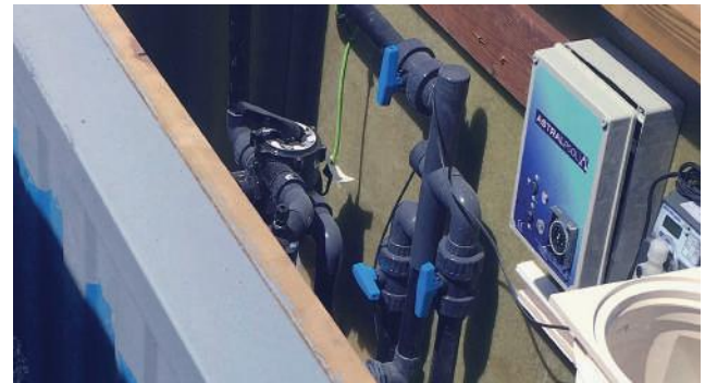
Installation technique dans local (1m x 2,5m)
